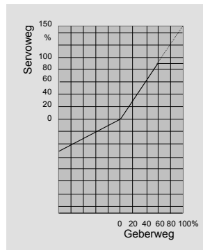
Die Abb. zeigt bei einer Wegeinstellung von + 150% die Wegbegrenzung des Servos auf 90%.
